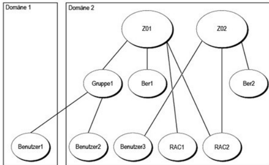
Abbildung 9-3. Active Directory-Objekte von RAC in mehreren Domänen einrichten
