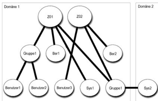
Abbildung 9-4. Active Directory-Objekte von Server Administrator in mehreren Domänen einrichten
